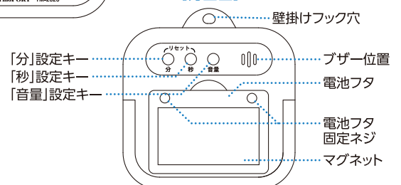
【背面図】
